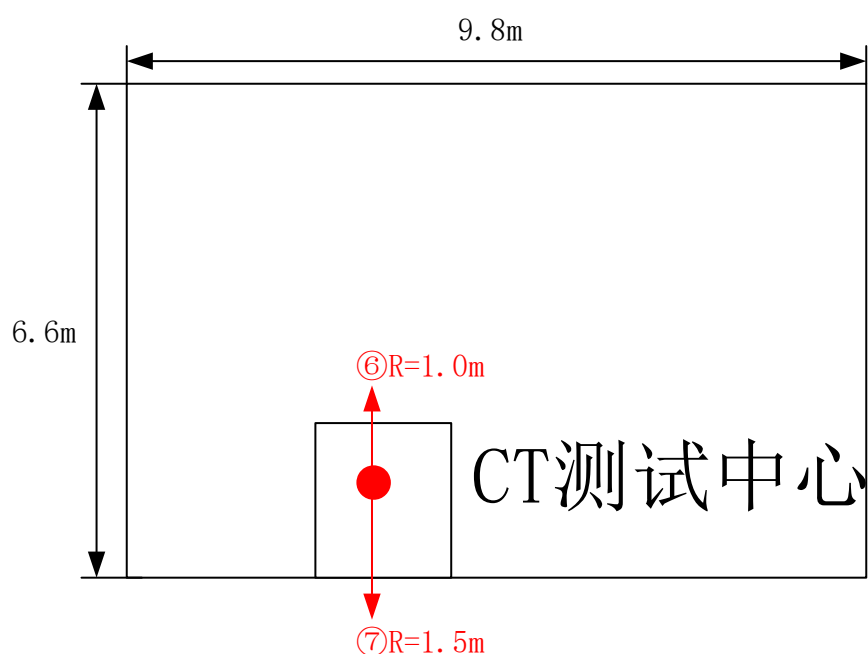
图 11-2.2 关注点分布示意图（立面）
