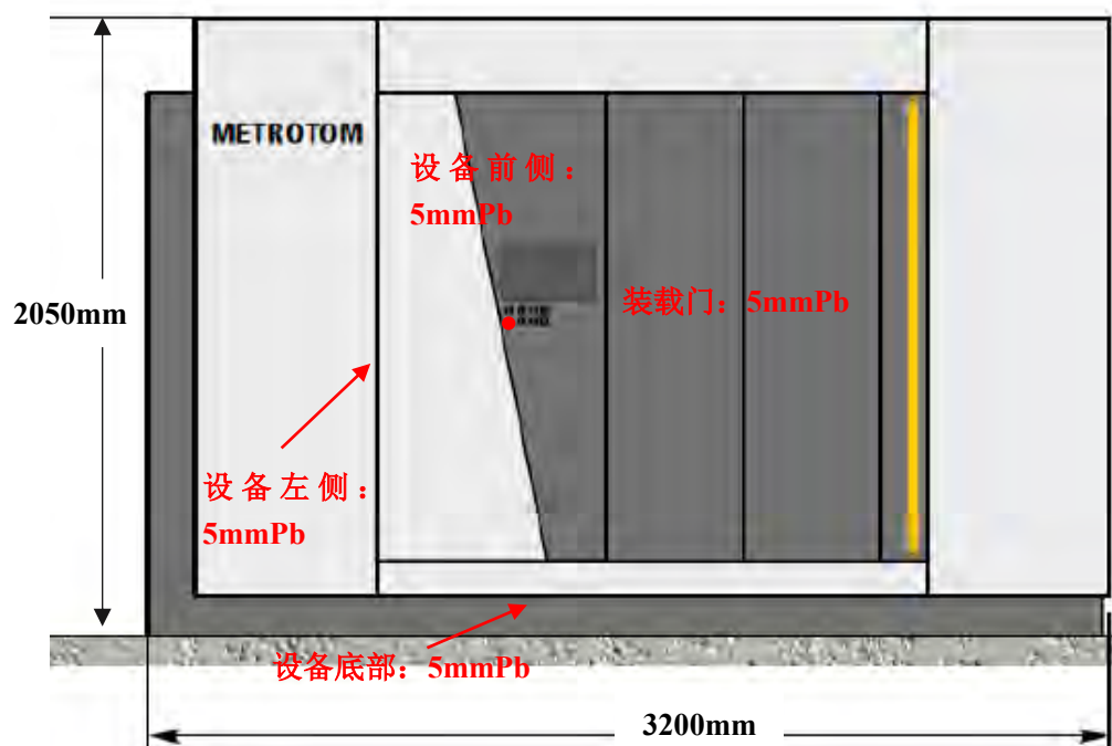
图 10-1 工业 CT 正视图
