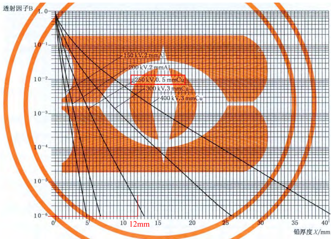
图 11-3 X 射线穿过铅的透射因子
