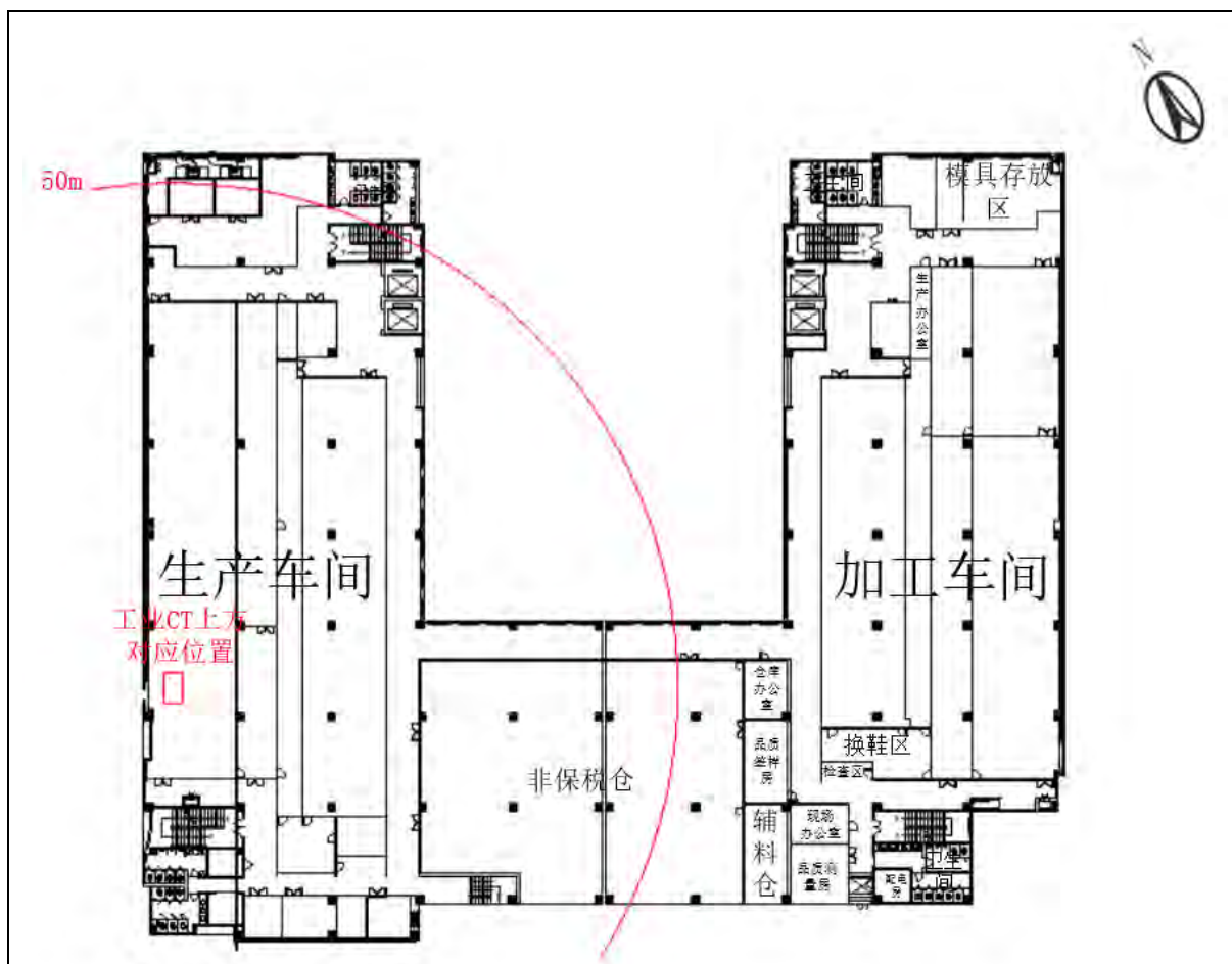
图 1-4 J 栋厂房 2 楼平面布置图
