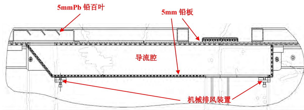
图 10-5 排风口屏蔽设计图
