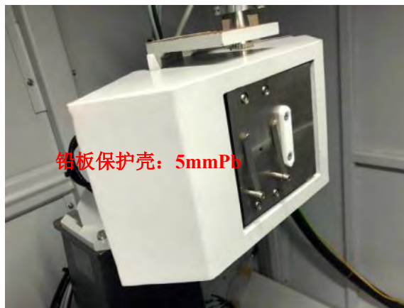
图 10-4 射线发生器铅保护外壳设计图
