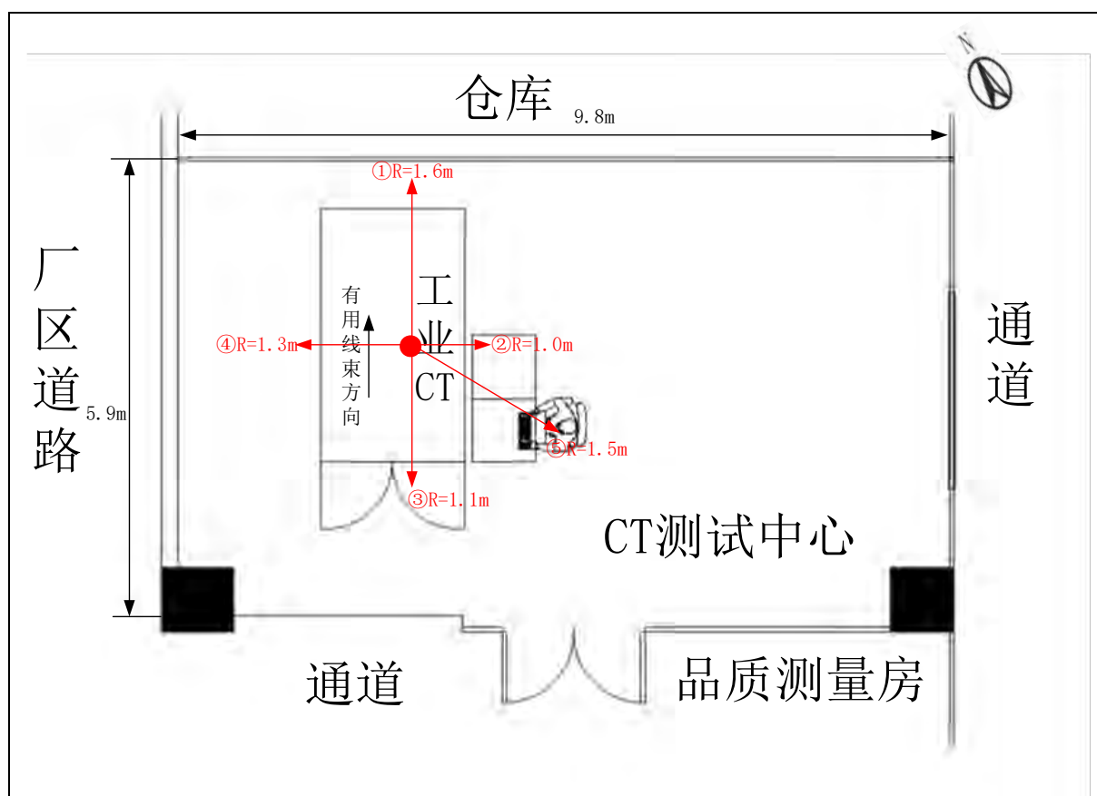
图 11-2.1 关注点分布示意图（平面）
