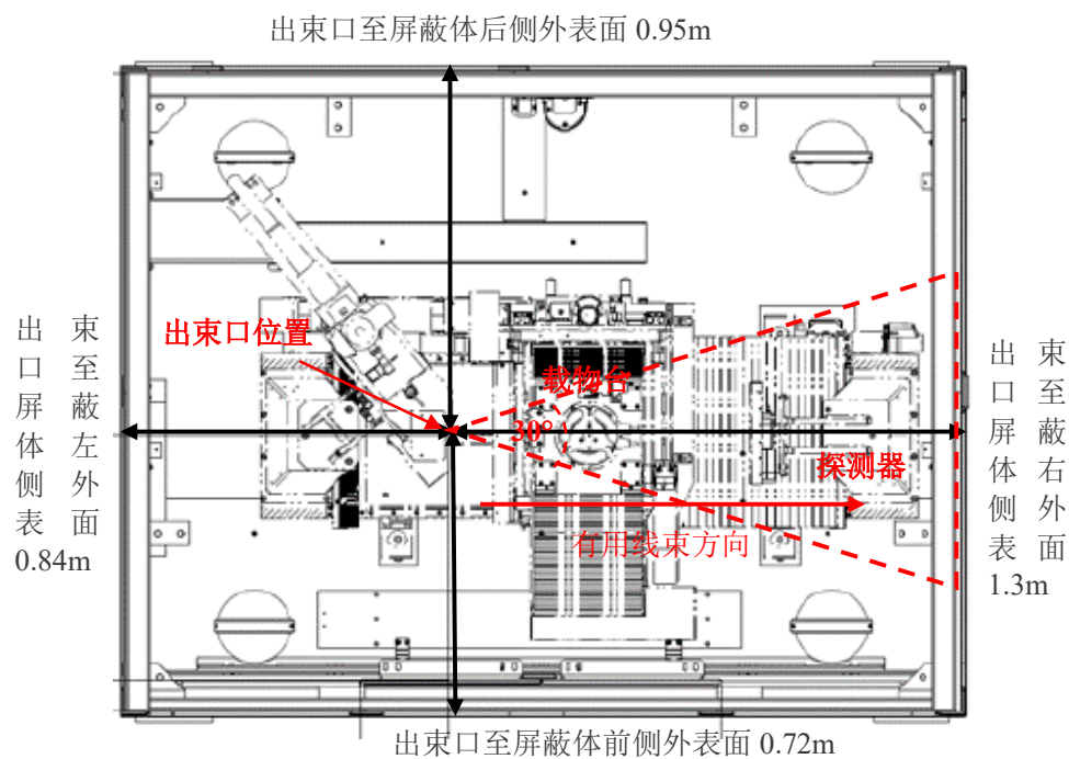
图 11-1.2 射线源分布示意图 (俯视图)
