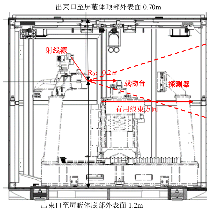
图 11-1.1 射线源分布示意图 (正视图)
