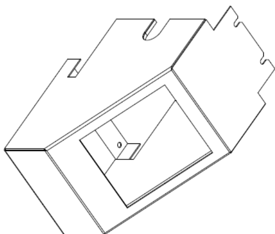
图 10-4 射线发生器铅保护外壳设计图
