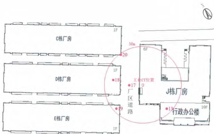
项目周边 50m 范围检测布点图
